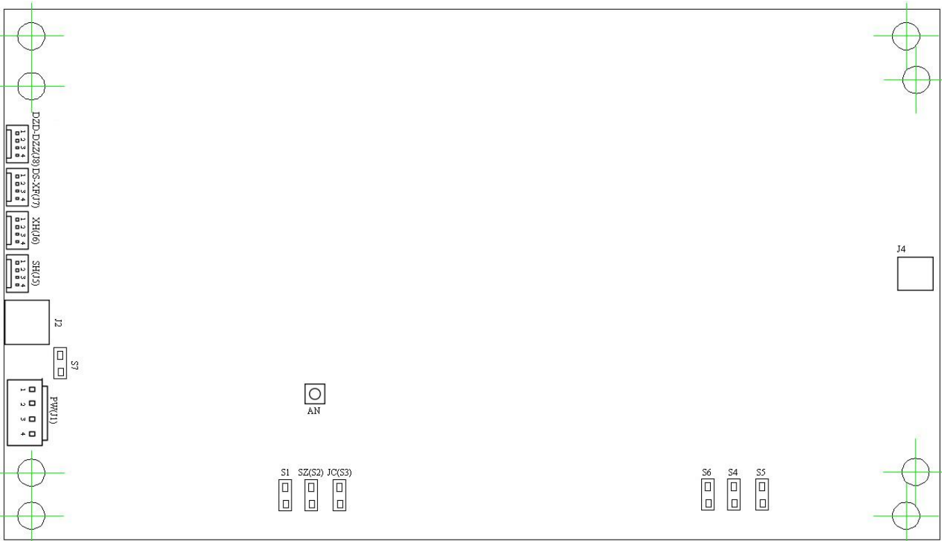
背面尺寸图
