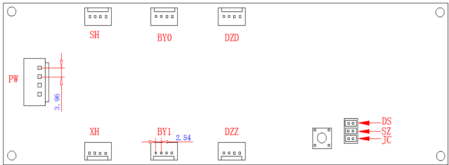
背面尺寸图
