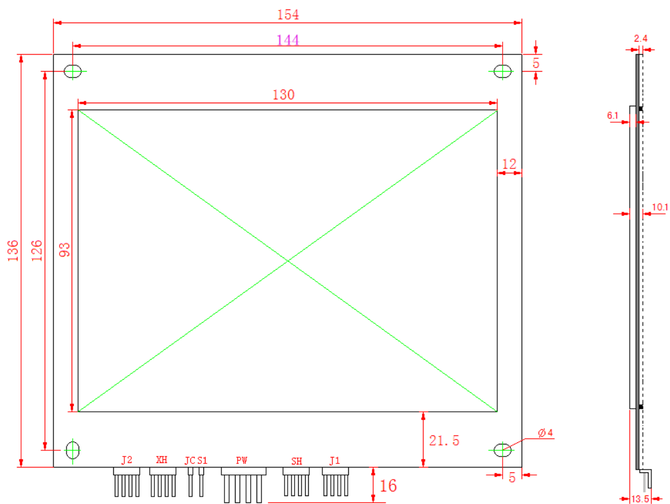
正面尺寸图
