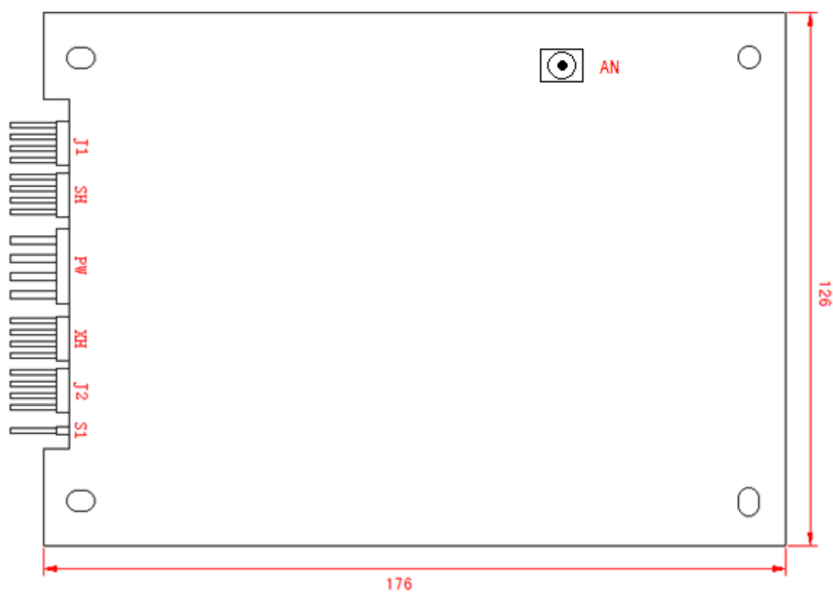
背面尺寸图
