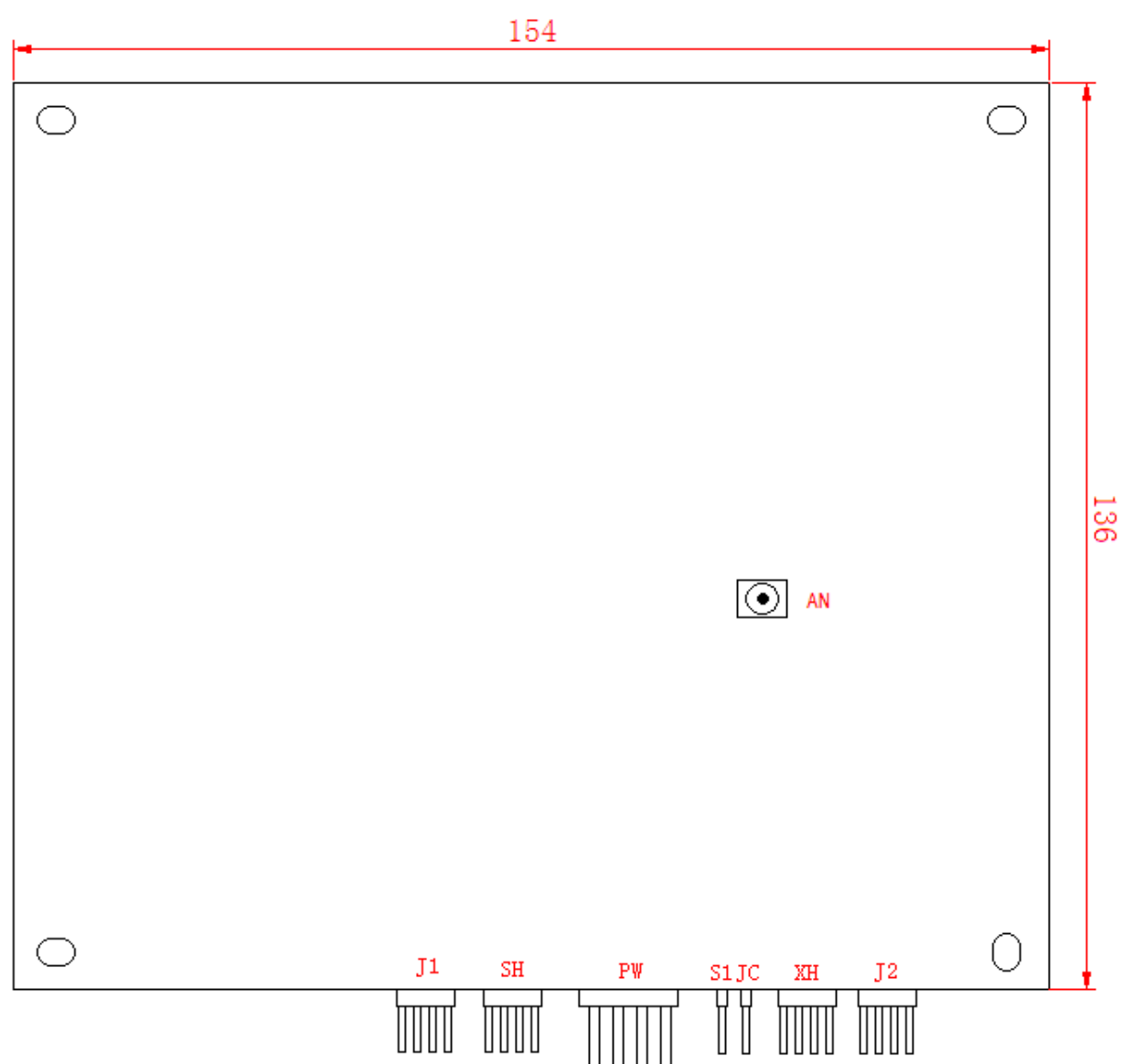
背面尺寸图
