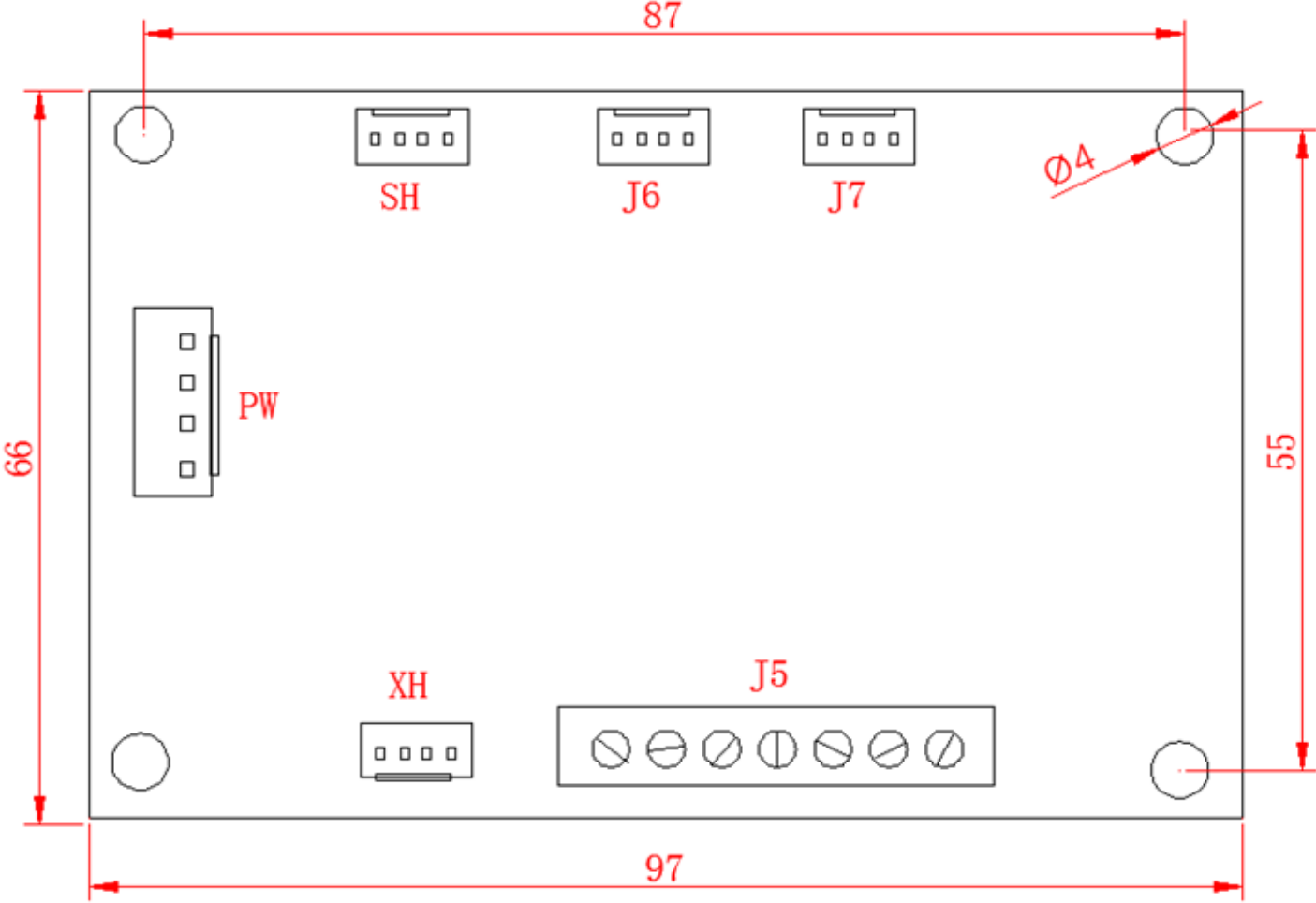
正面尺寸图
