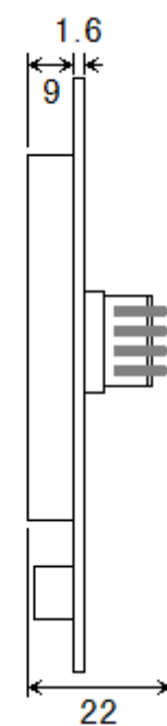
侧面尺寸图
