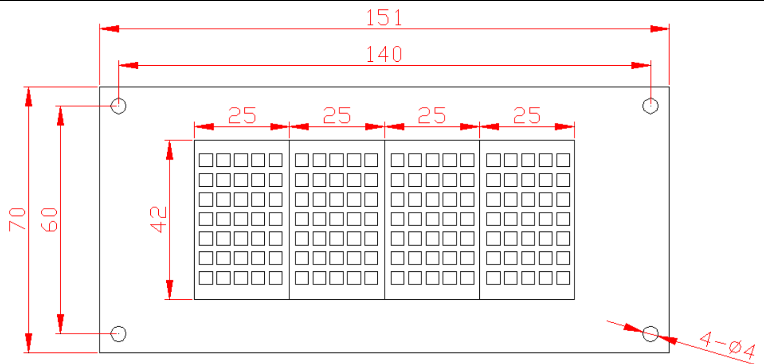
正面尺寸图
