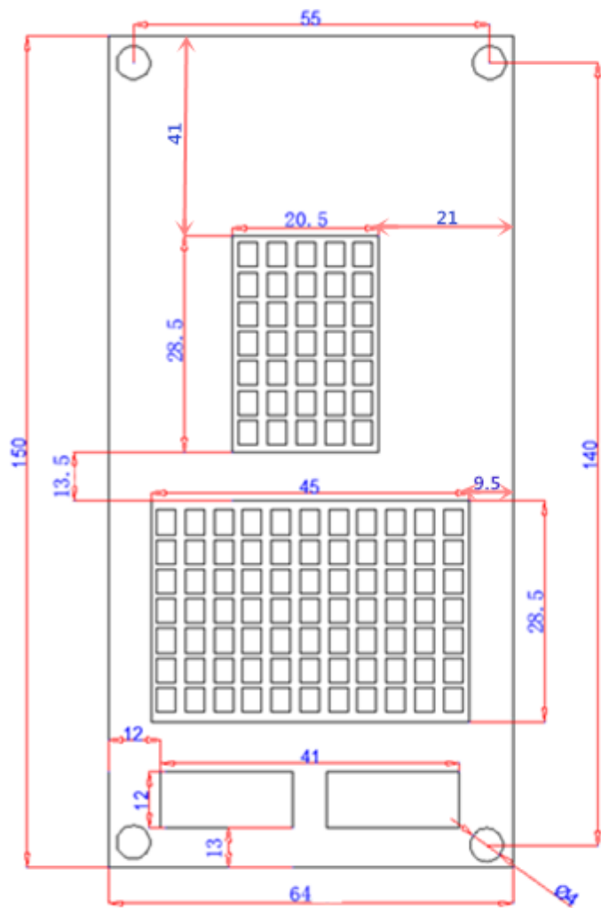
正面尺寸图
