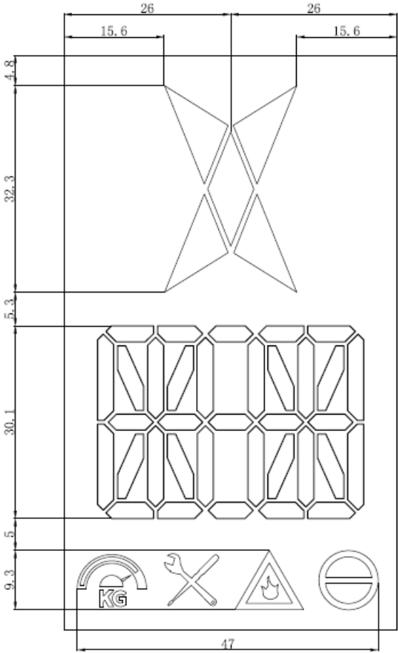
屏显尺寸图
