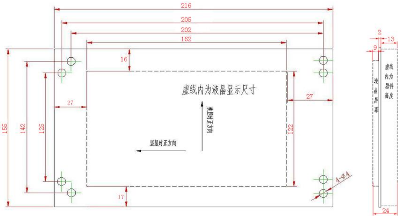
正面尺寸图
