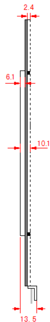
侧面尺寸图
