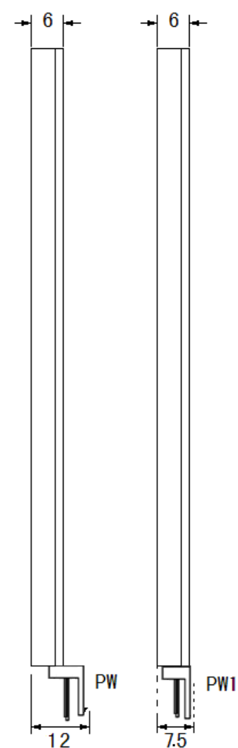
侧面尺寸图
