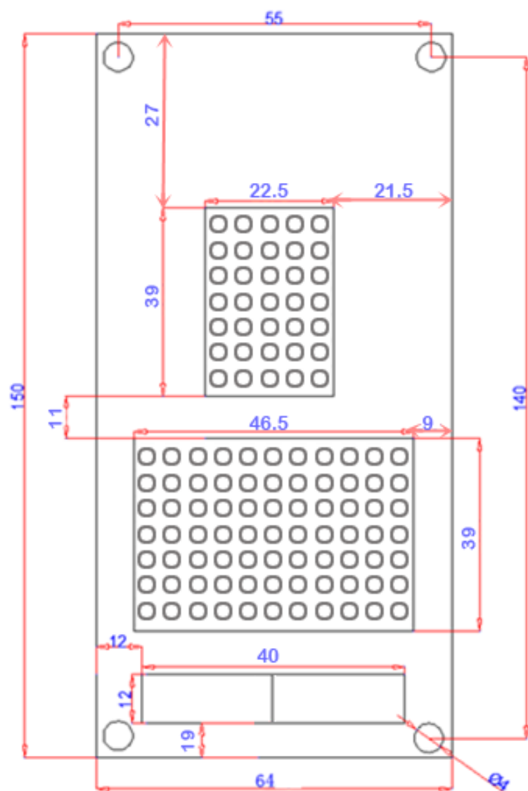
正面尺寸图
