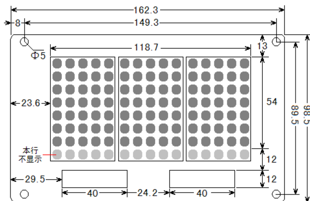
正面尺寸图
