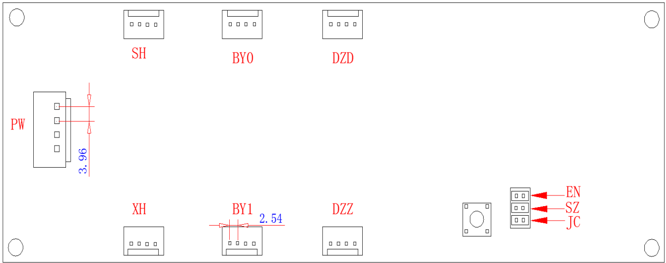
背面尺寸图
