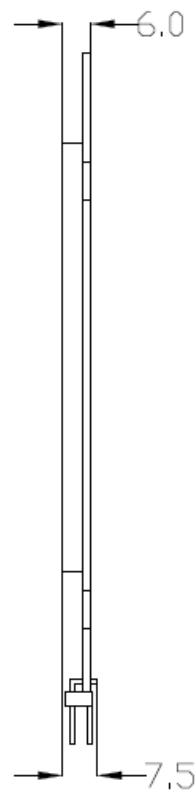
侧面尺寸图
