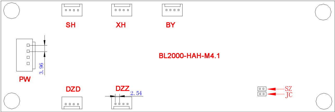
BL2000-HAH-M4.1 背面尺寸图
