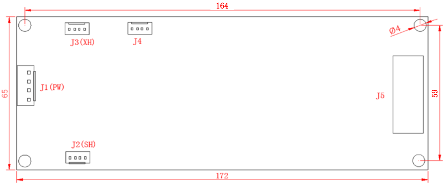
正面尺寸图
