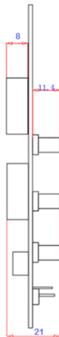
侧面尺寸图
