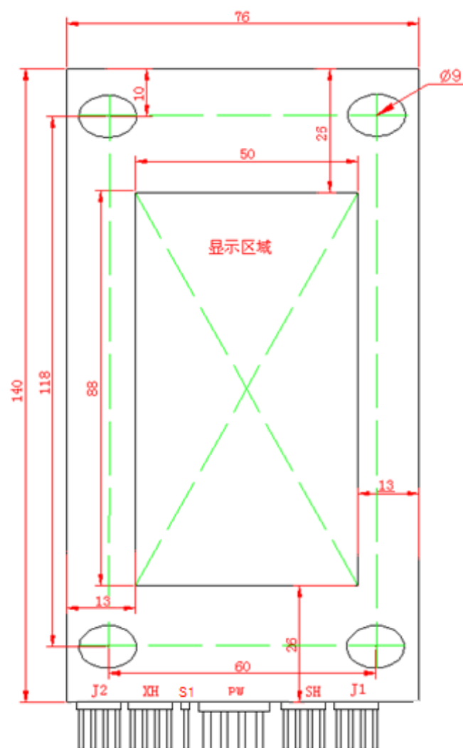
正面尺寸图
