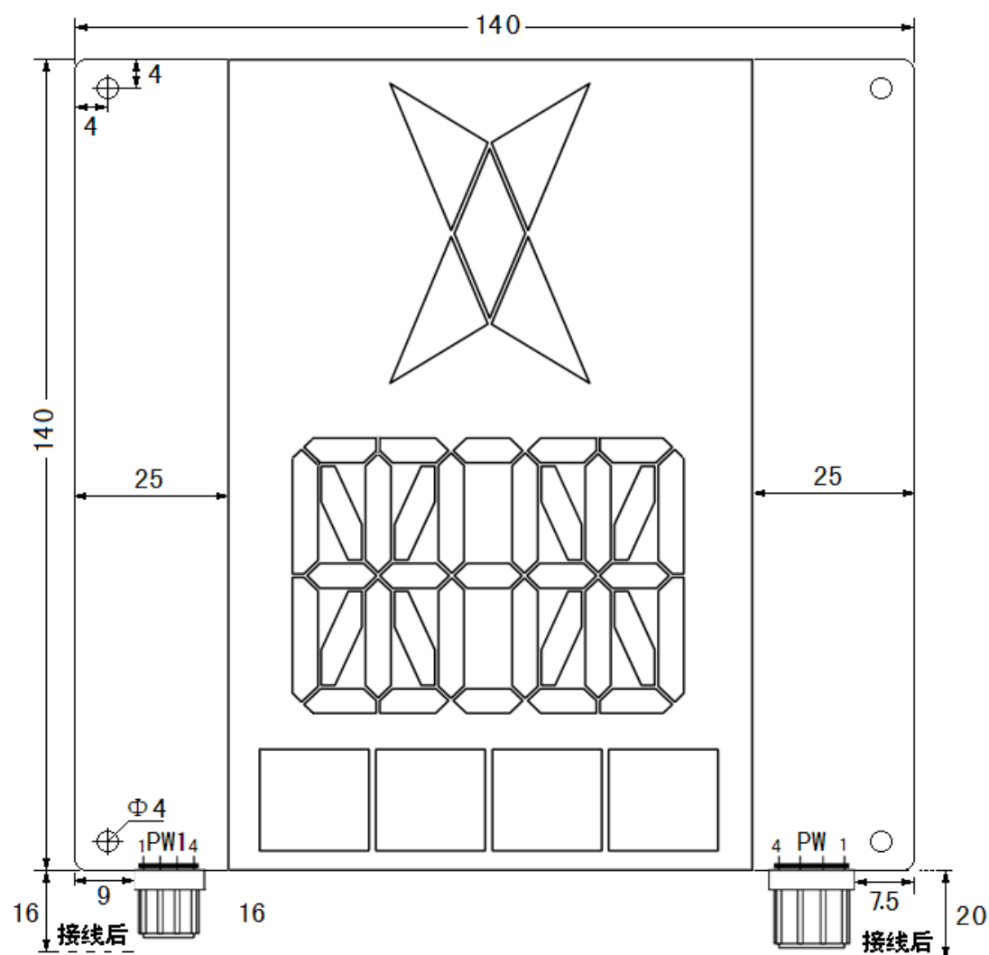
正面尺寸图
