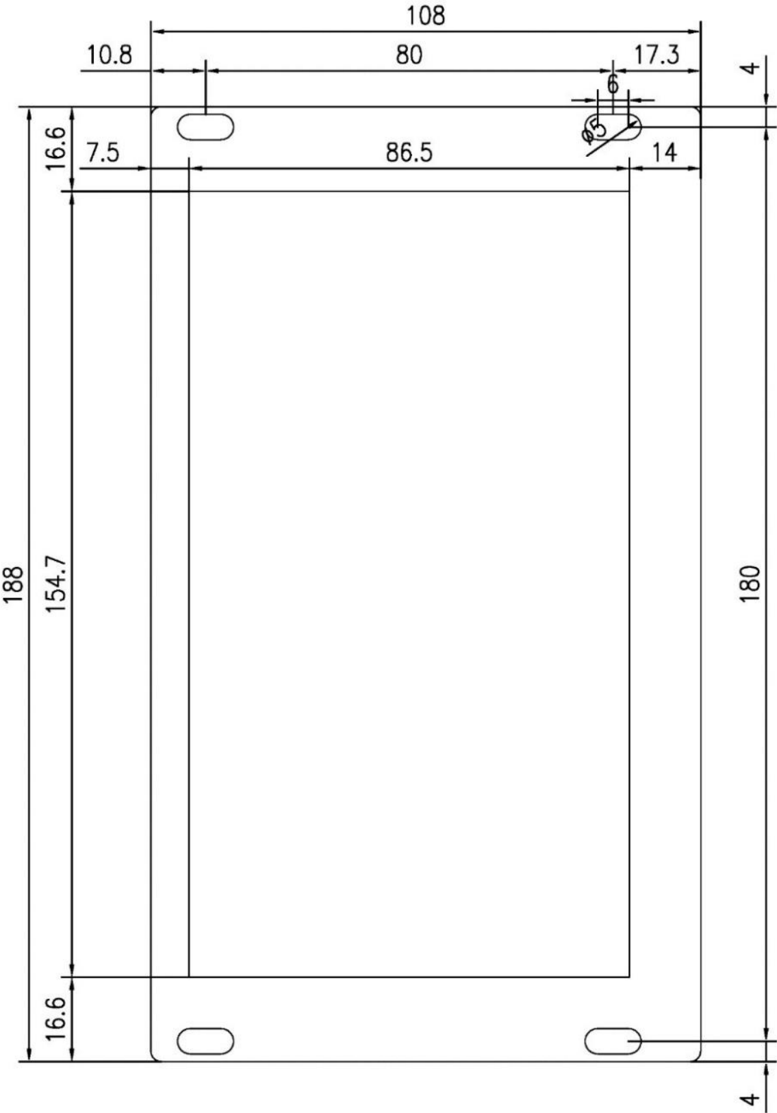
正面尺寸图
