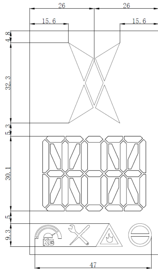
屏显尺寸图
