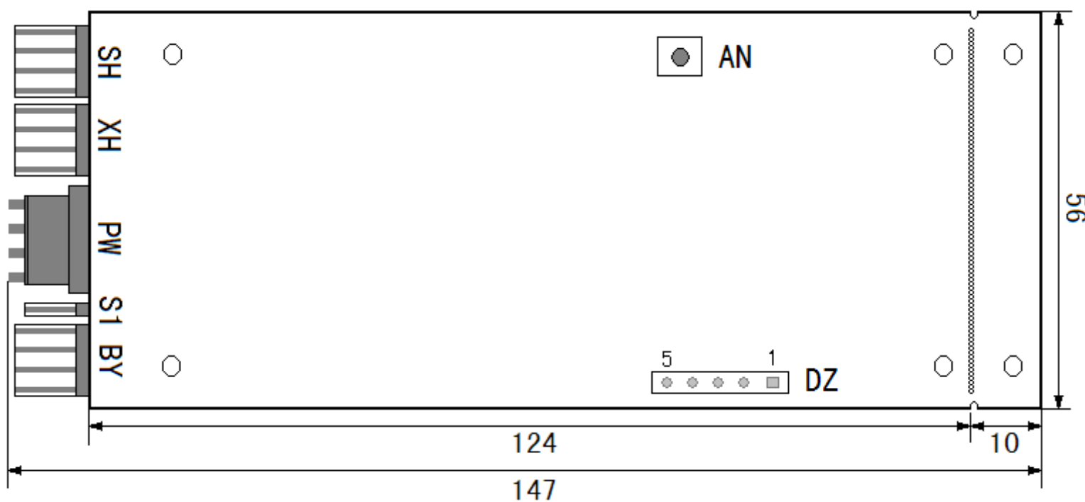
背面尺寸图
