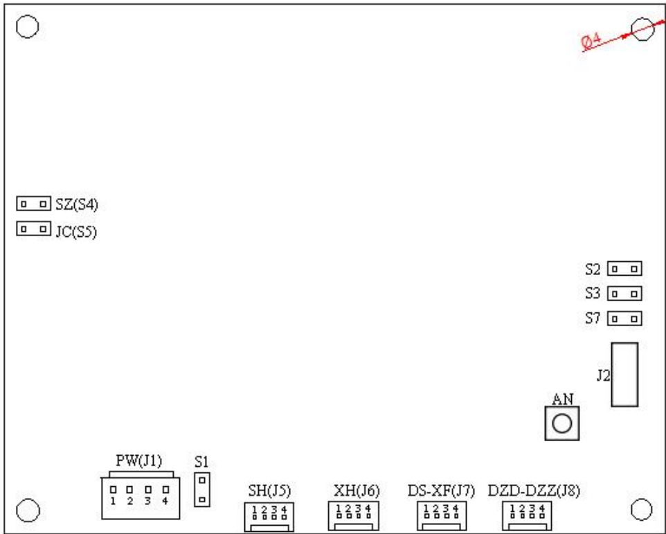
背面尺寸图
