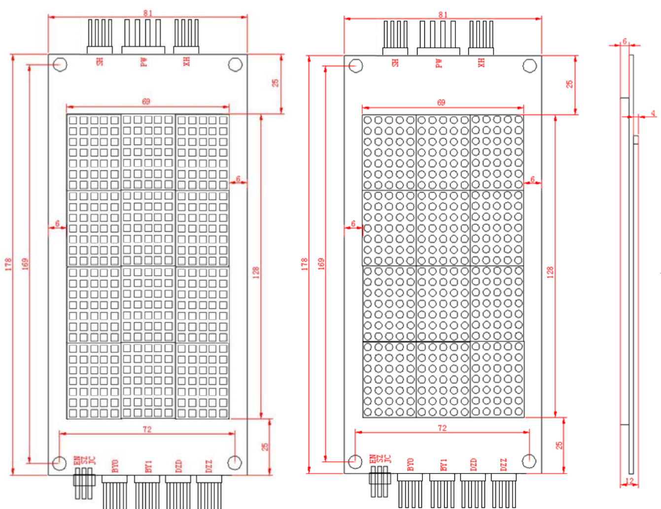
正面尺寸图
