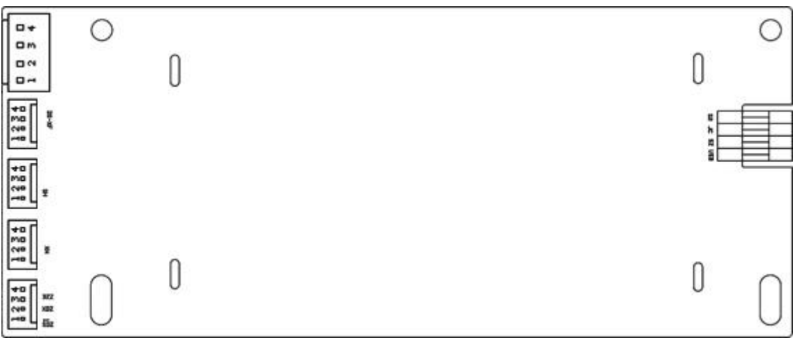
背面尺寸图
