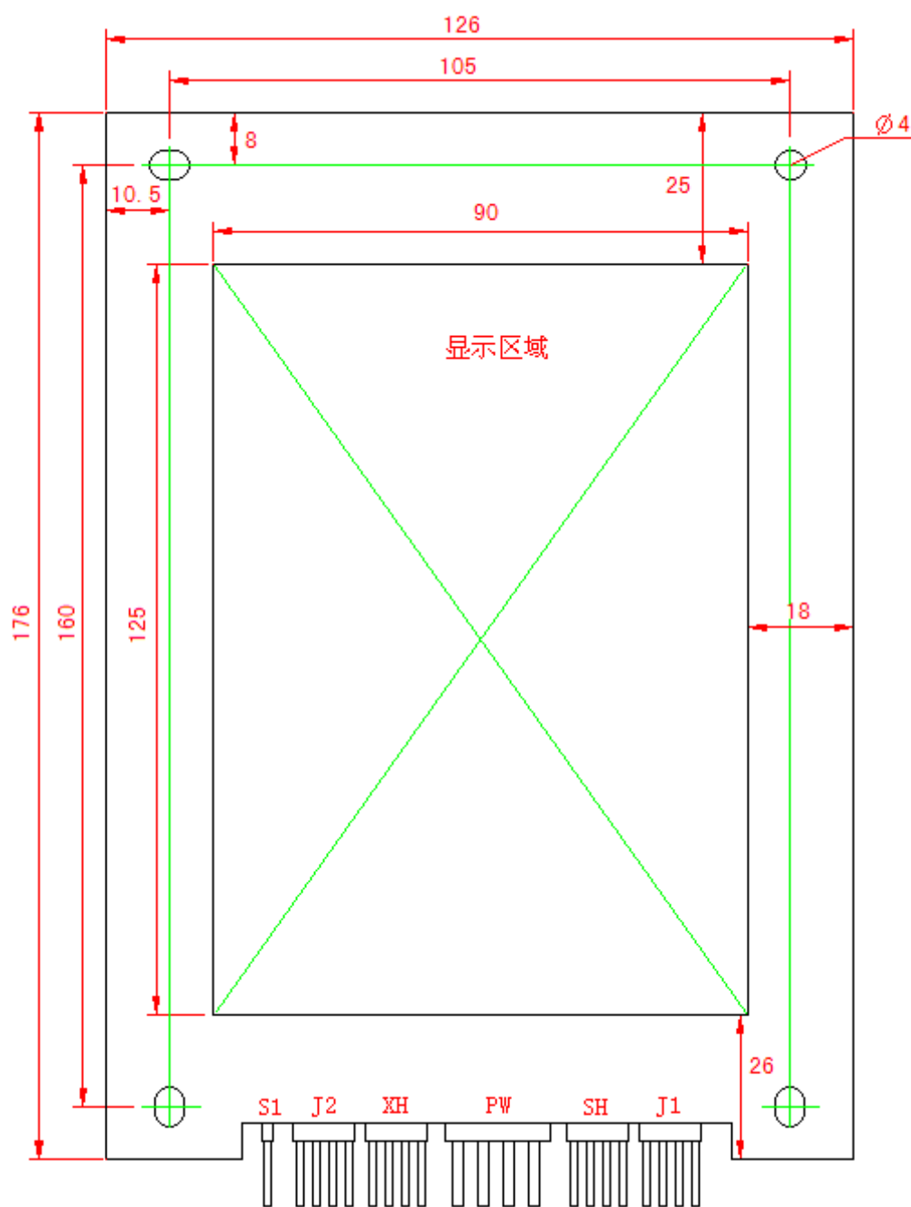
正面尺寸图
