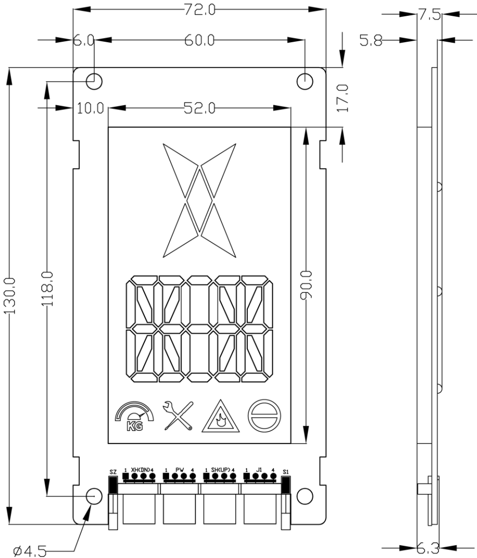
正面尺寸图
