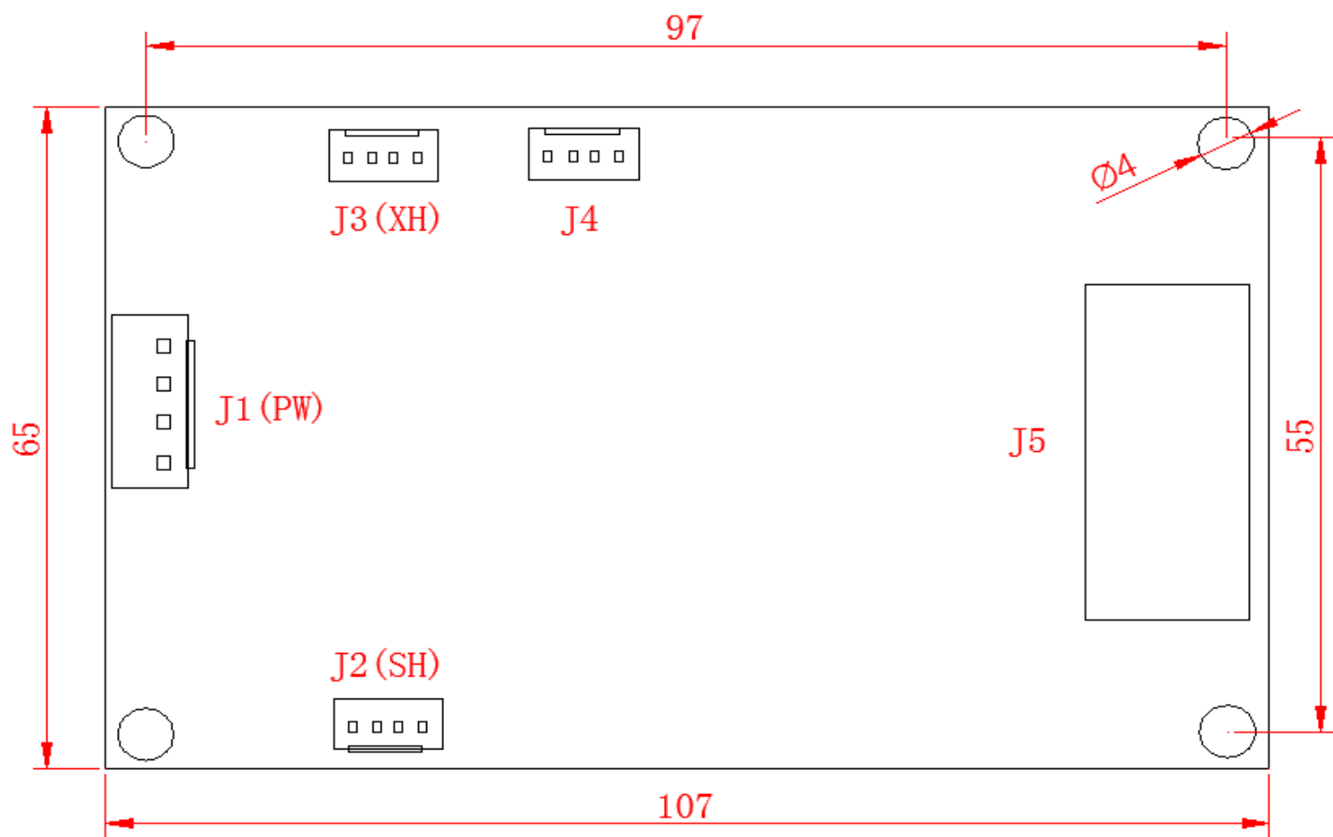
正面尺寸图
