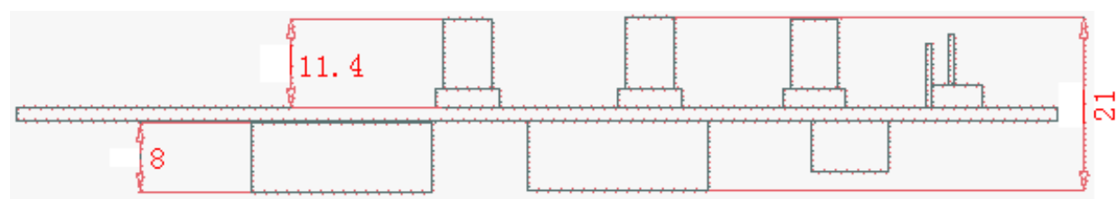
侧面尺寸图
