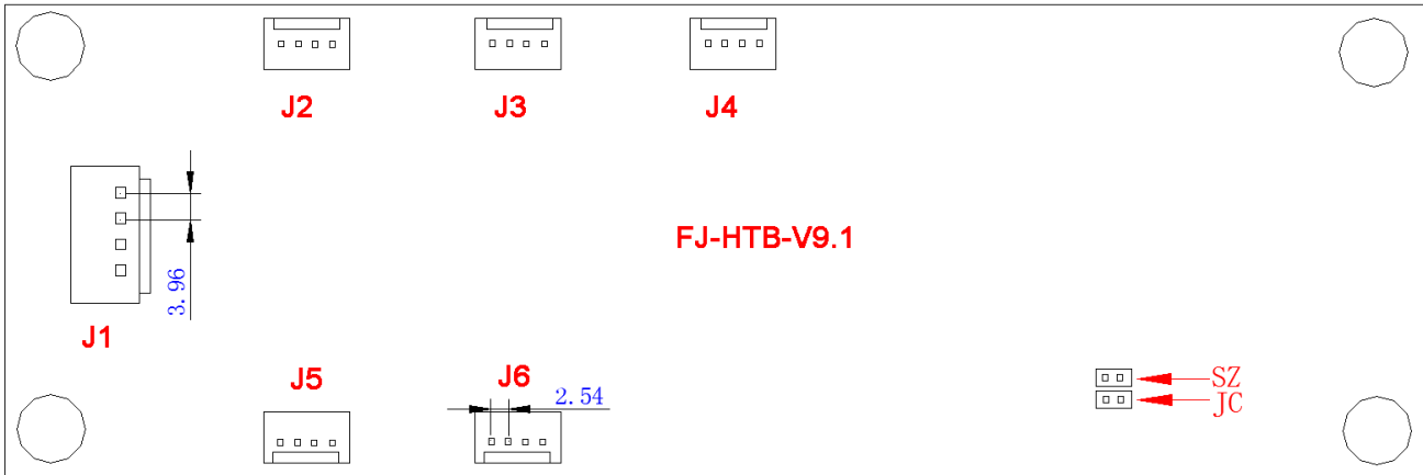
FJ-HTB-V9.1 背面尺寸图
