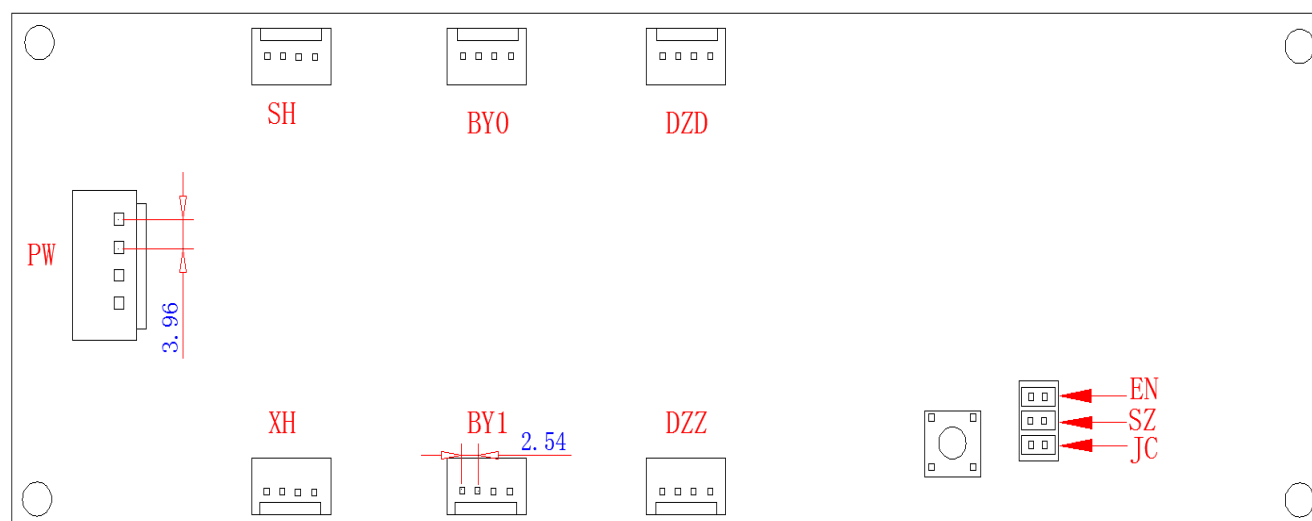
背面尺寸图
