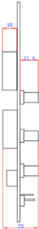
侧面尺寸图
