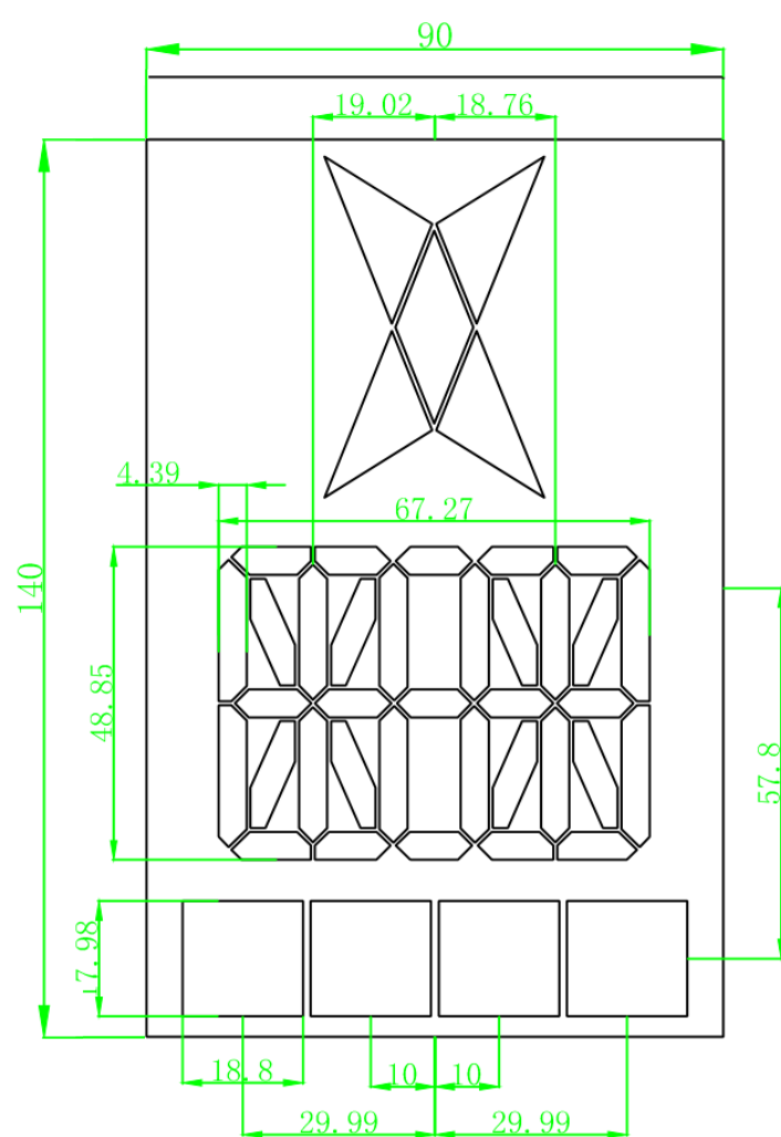
屏显尺寸图
