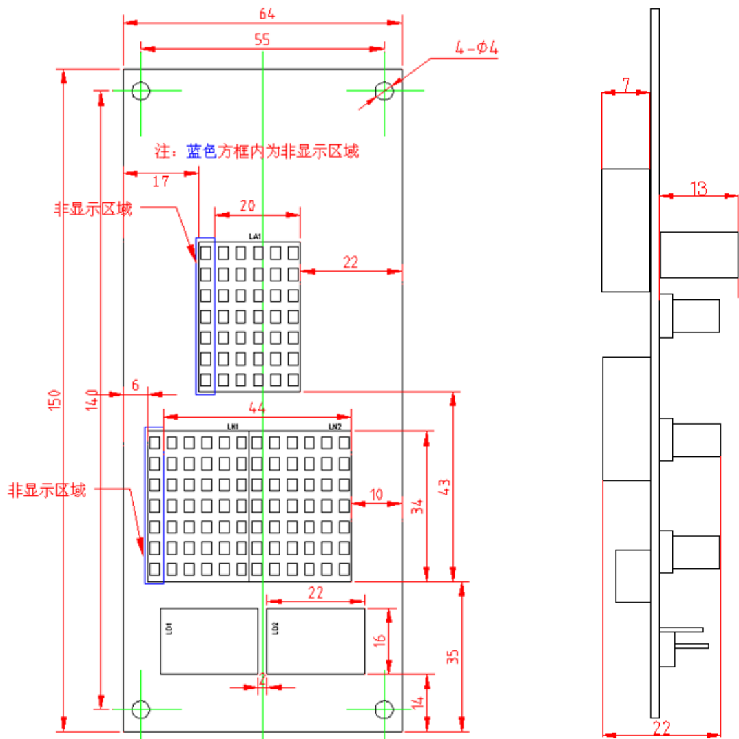
正面尺寸图
