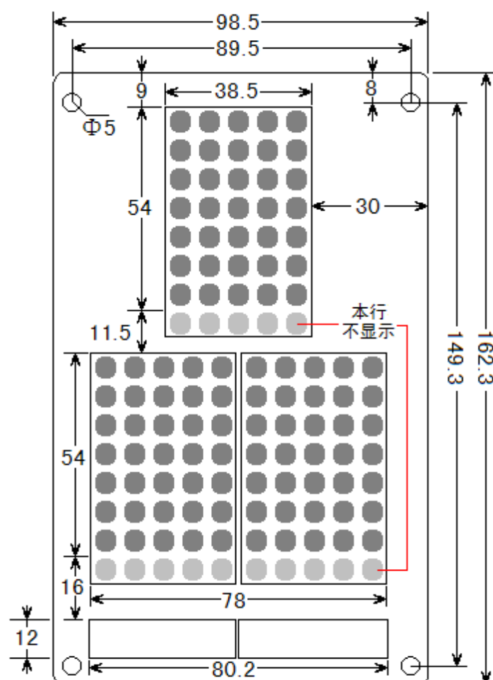
正面尺寸图
