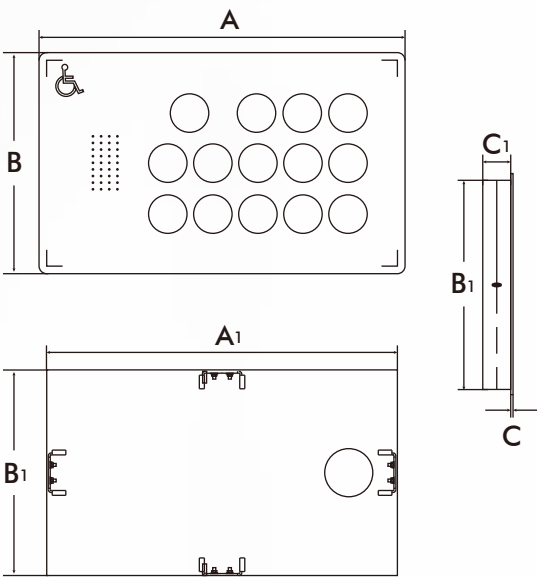
尺寸图
