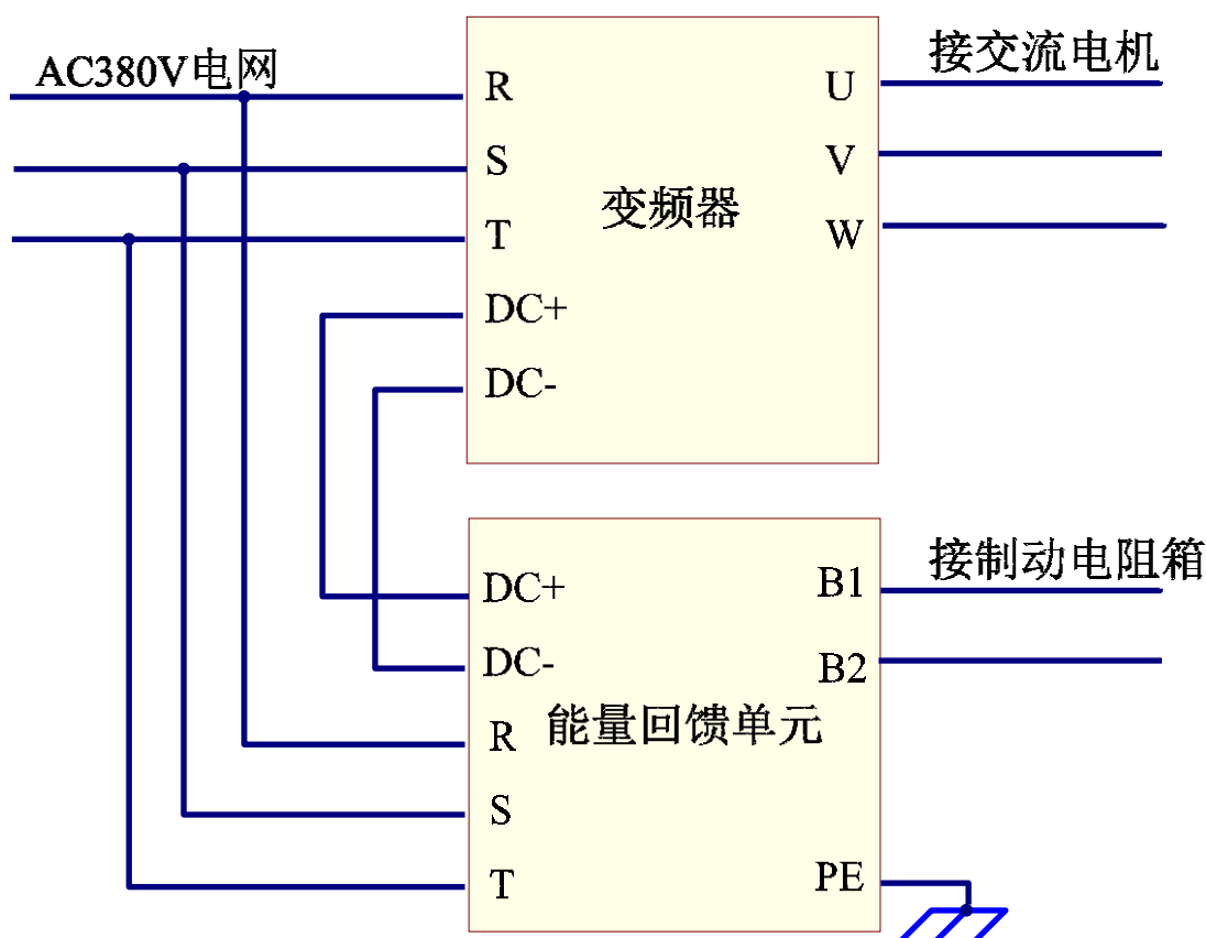
图 3.1 (b) 主回路结构示意图 (110KW)
