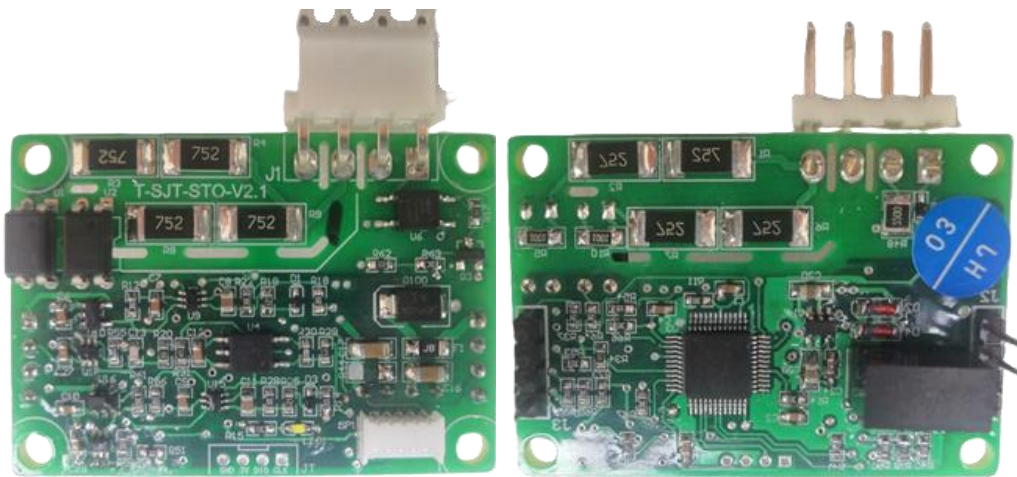
图 F24.1 SJT-STO-V2.1 产品外观
