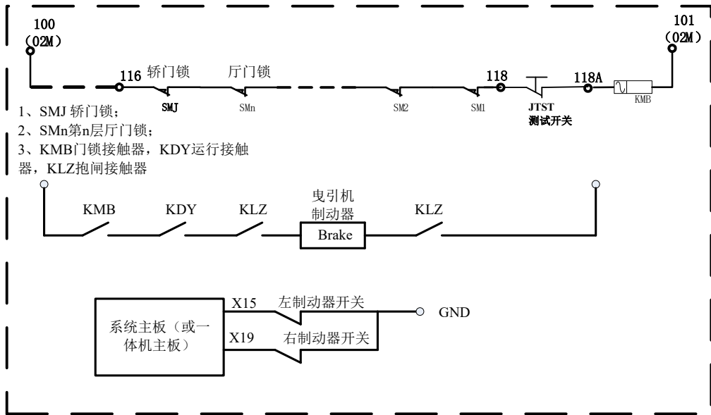
图 F10.1 制动器控制接线示意图
