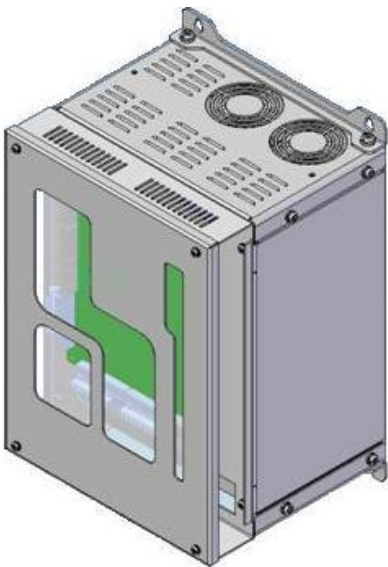
图 2.10 带铁面板安装外形图
