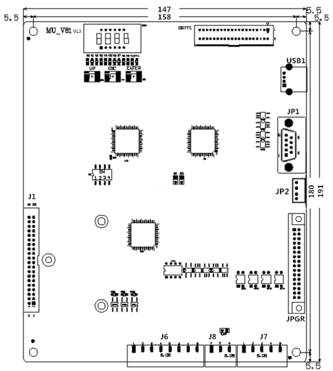
图 3.5 主控板端子排列尺寸图
