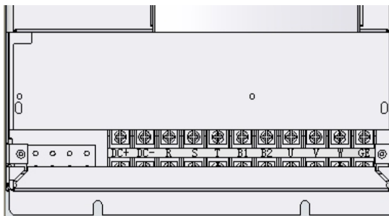
图 3.3 主回路端子排列示意图
