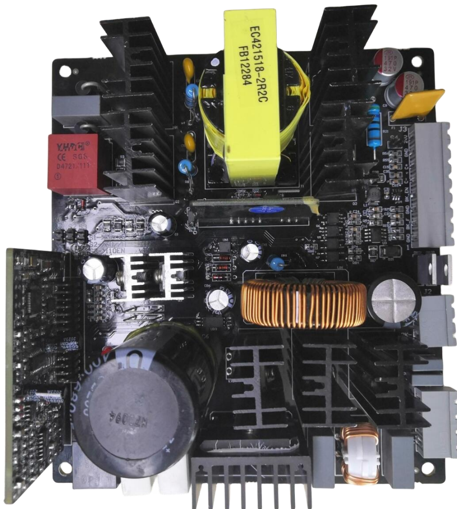
图 11.5 SJT-POBK-V1.3 抱闸电源板实物图
