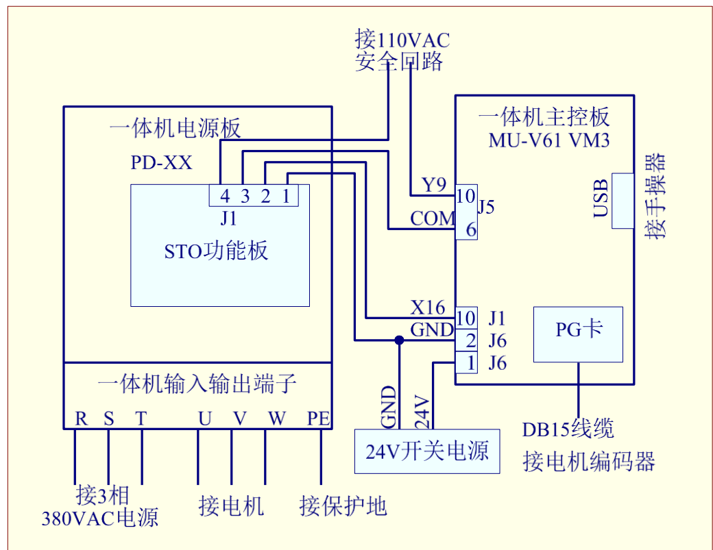
图 F24.4 SJT-STO-V2.1 系统接线原理图
