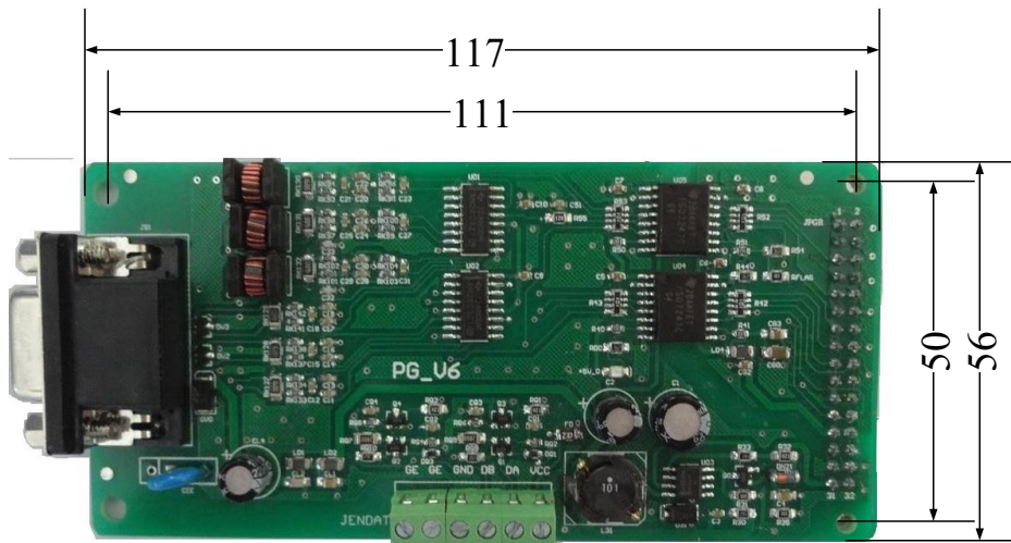
图 3.11 PG_V6 卡外型示意图
