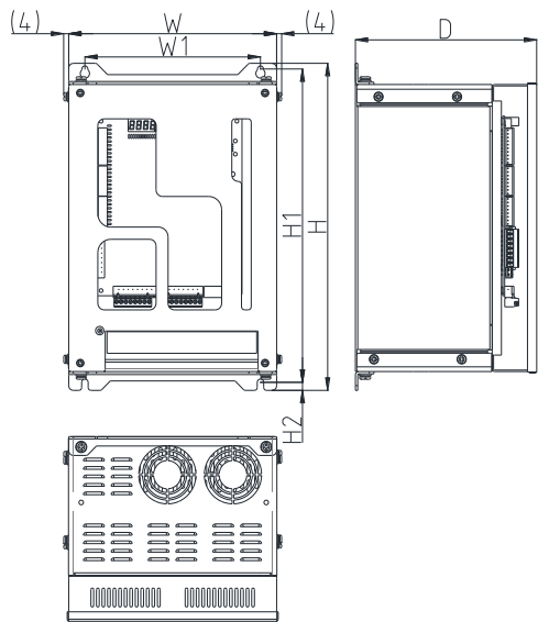
图 2.9 带铁面板安装尺寸示意图
