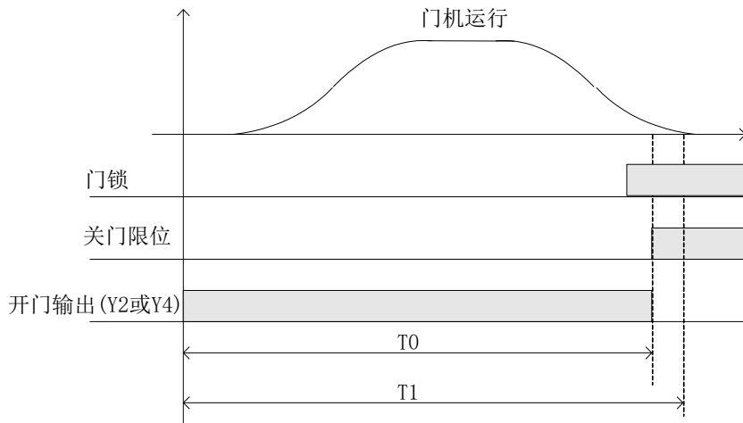
图 6.8 关门时序图
