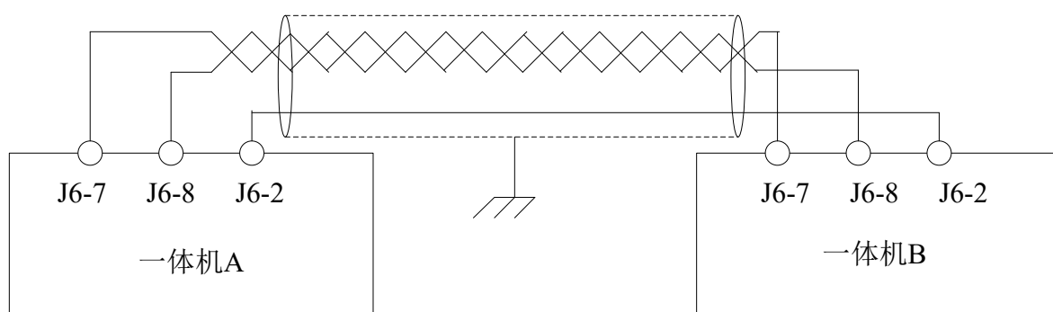
图 6.9 并联连接示意图
