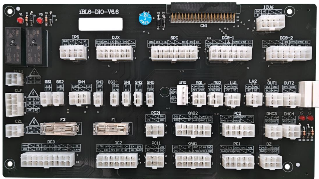
图 11.3 iBL6-DIO-V6.6 轿顶接口板实物图及尺寸图
