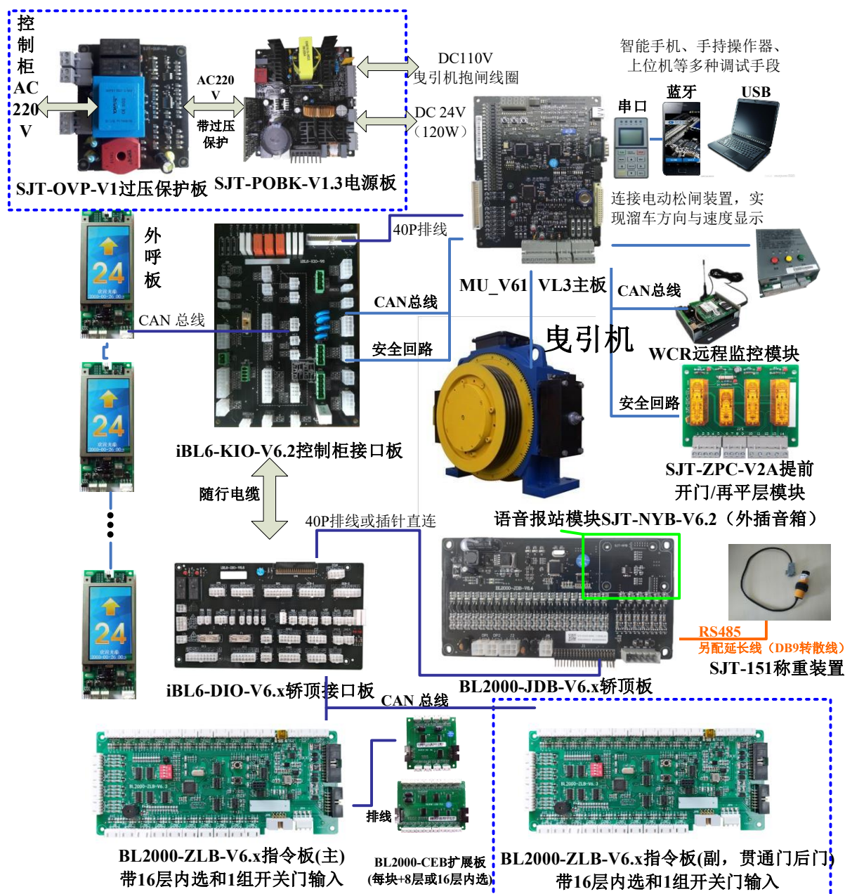
图 2.1 模块化一体机系统构成图
