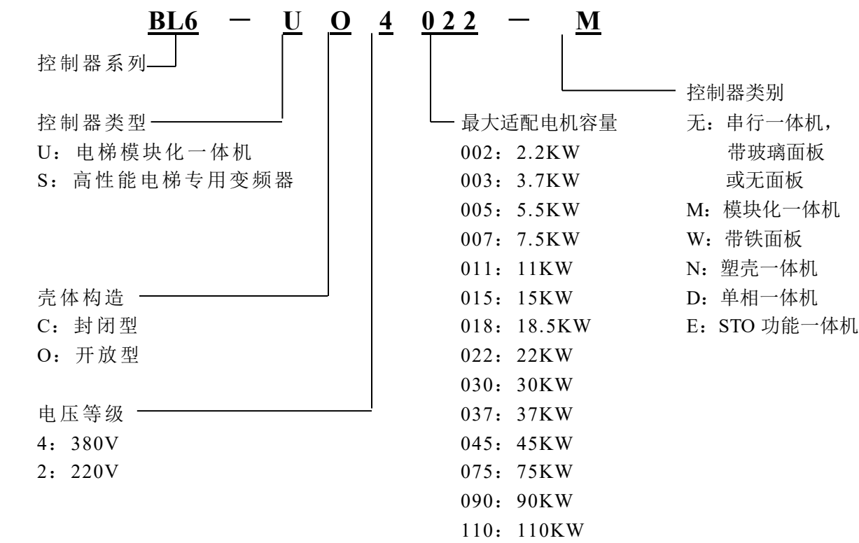
图 2.2 型号说明示意图
