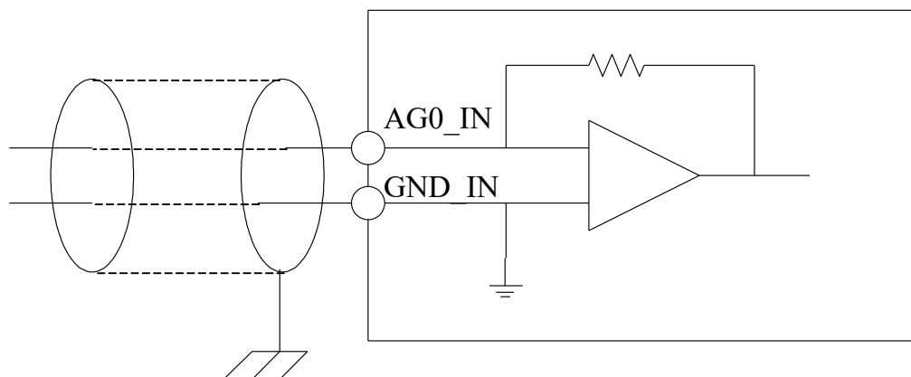
图 3.8 模拟输入原理及接线示意图
