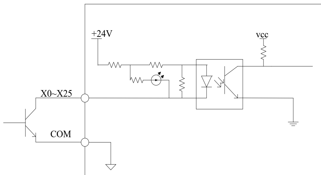
图 3.5 共发射极输入示意图
