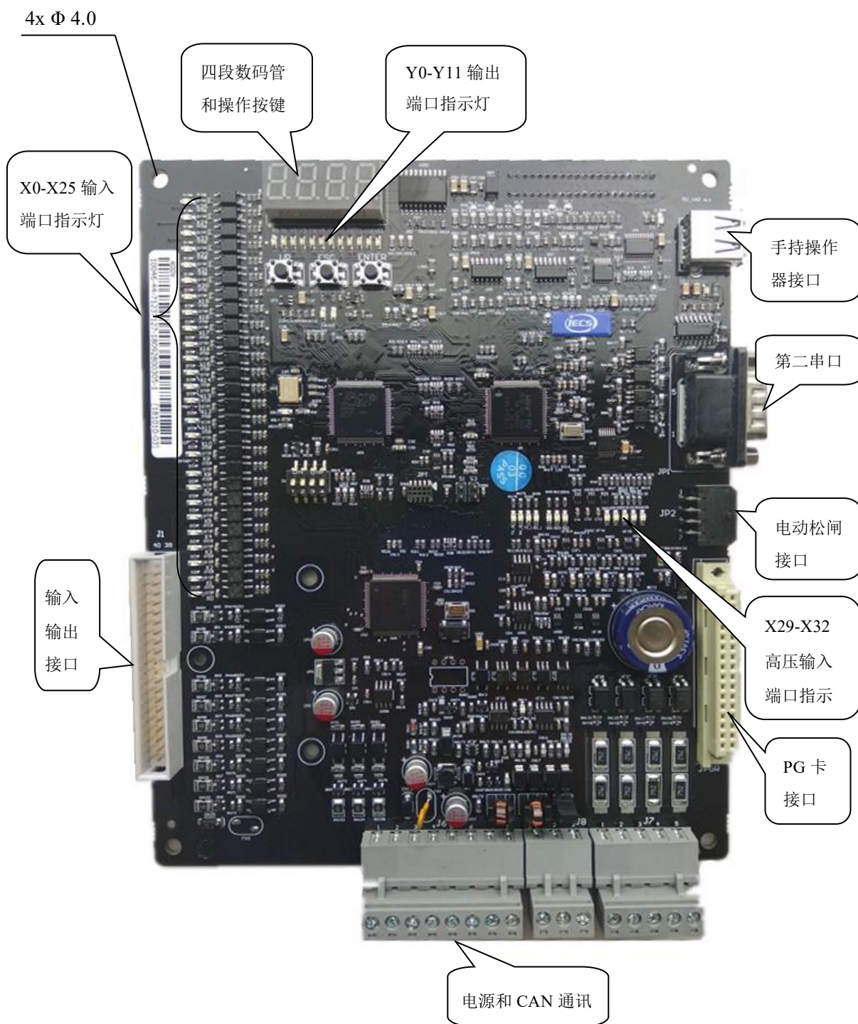
图 3.4 控制回路端子排列示意图
