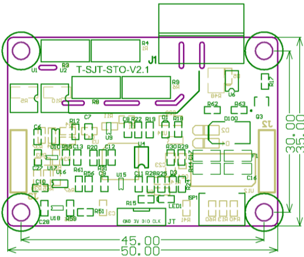
图 F24.2 SJT-STO-V2.1 产品尺寸（单位：mm）
