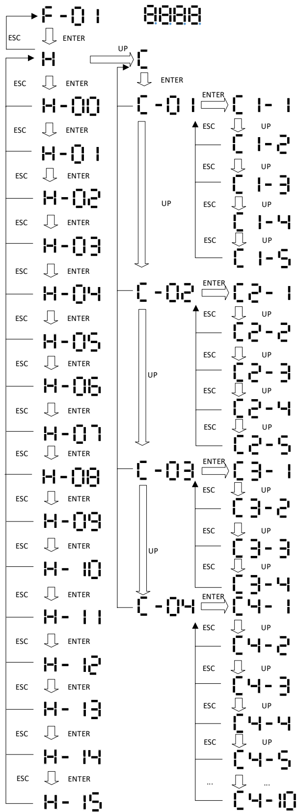
图 F7.3 主控板数码块与按键配合设置流程图（C 组）
