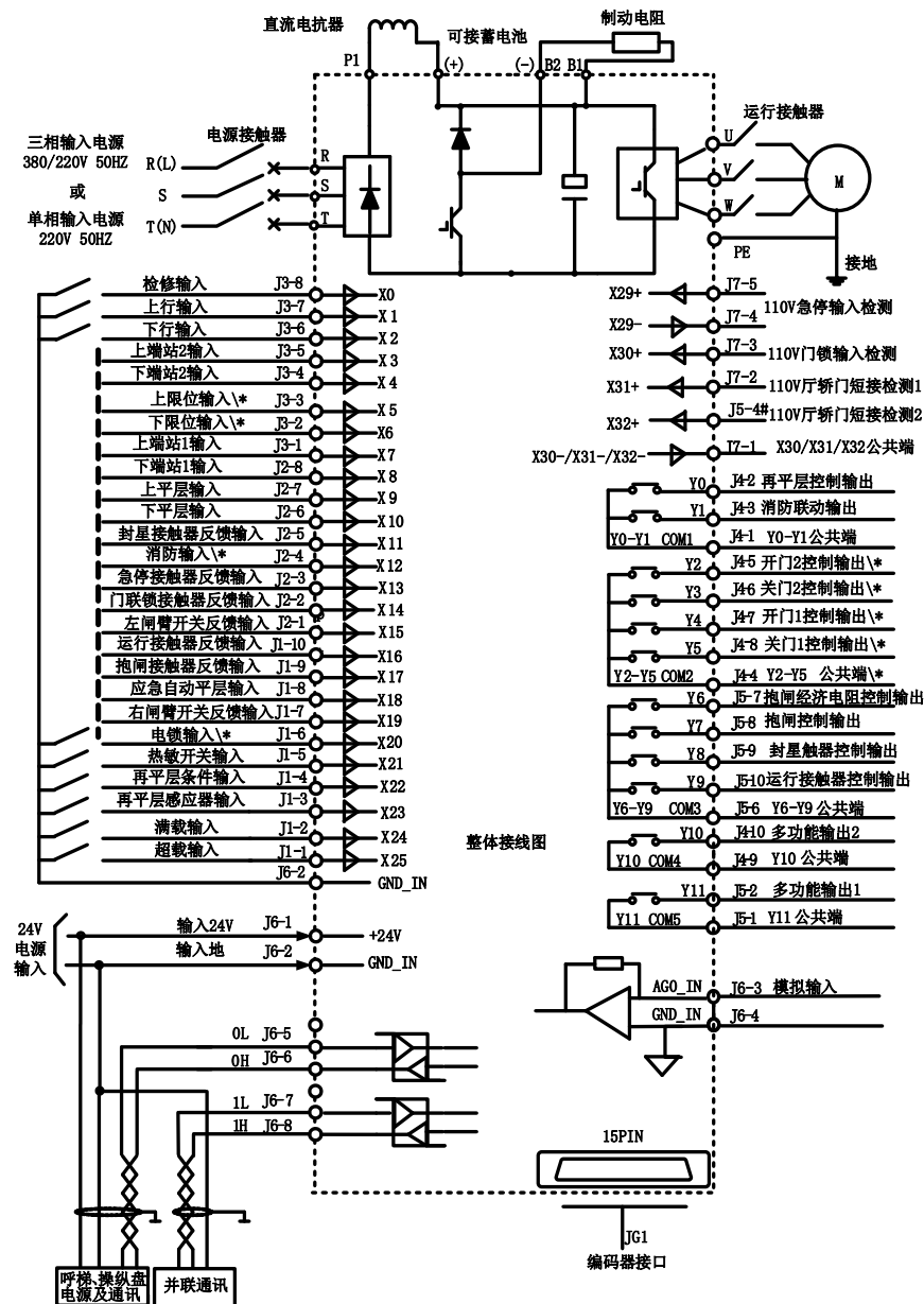
图 3.1 电梯模块化一体机接线示意图
