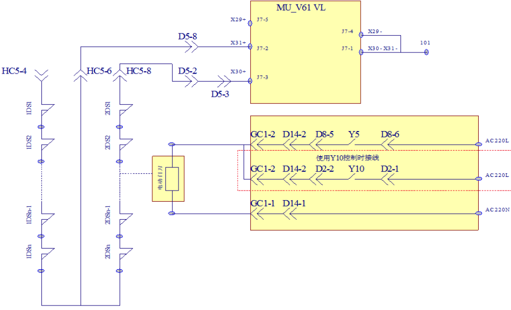
图F21.1 门锁回路示意图
