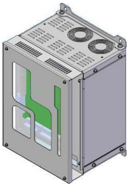
图 2.4 带铁面板安装外观图
