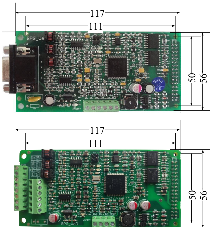
图 3.16 SPG_V6 / SPG_V6D 外型尺寸图
