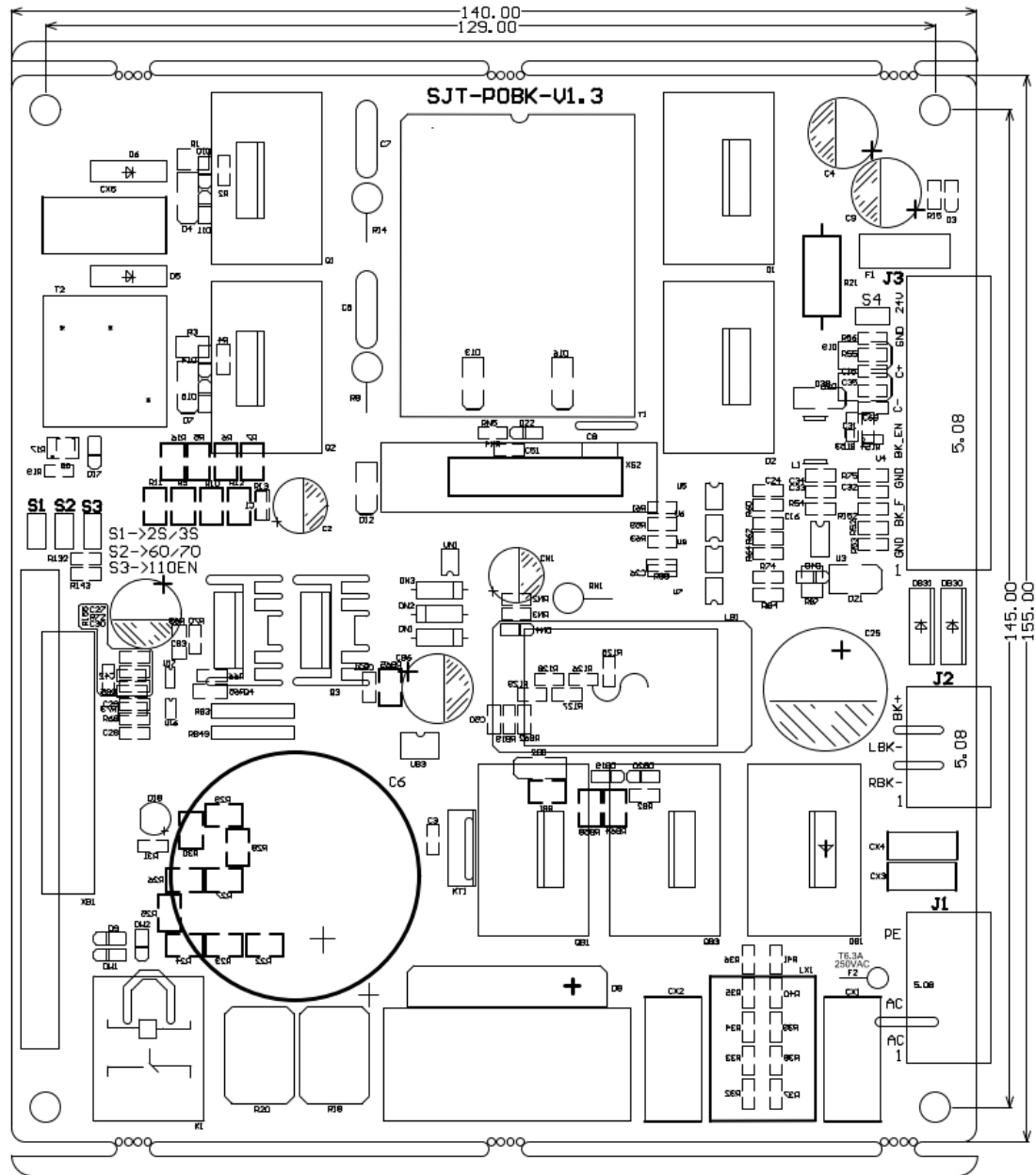
图 11.6 SJT-POBK-V1.3 安装尺寸图
