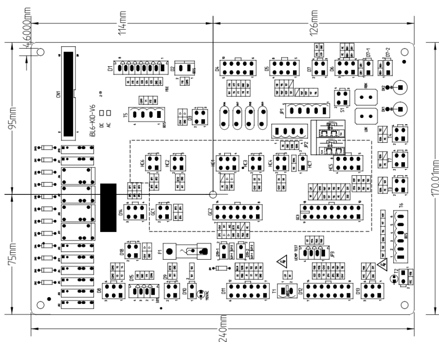
图 11.2 iBL6-KIO-V6.2 (x) 控制柜接口板器件位置及尺寸图
