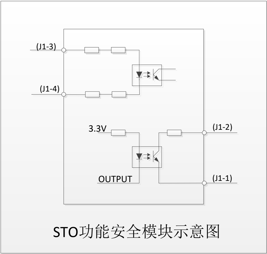
图 F24.3 接口电路示意
