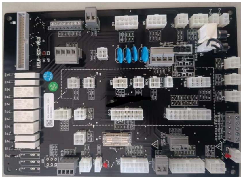
图 11.1 iBL6-KIO-V6.2 (x) 控制柜接口板实物图
