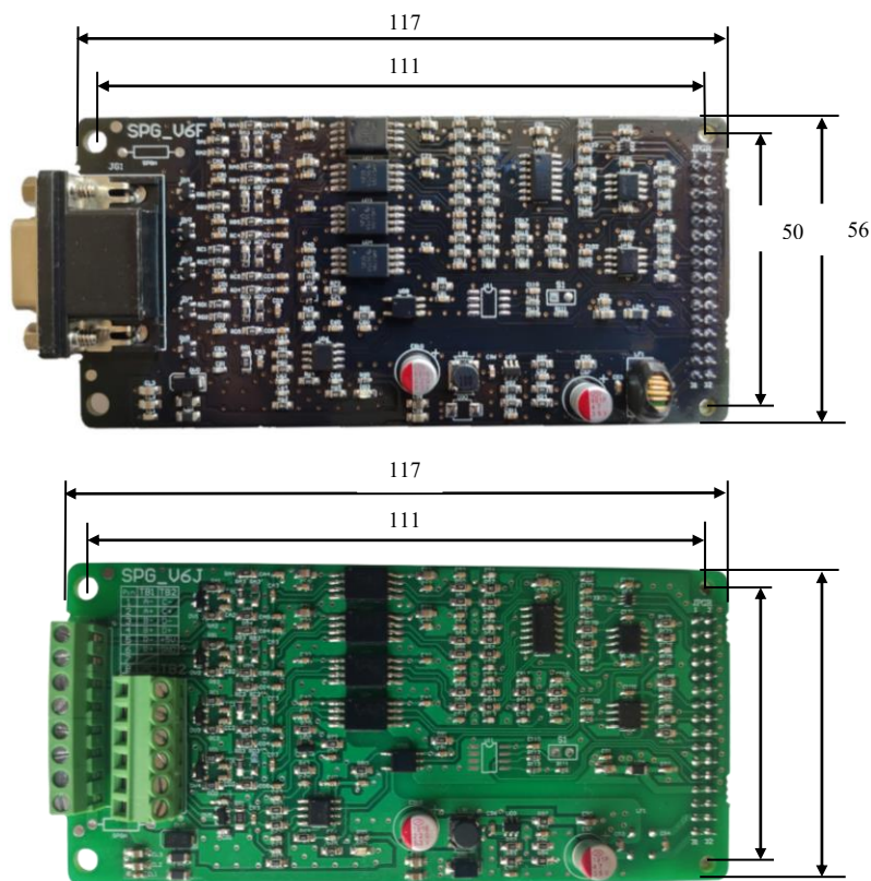
图 3.19 SPG_V6F / SPG_V6J 接口卡外型尺寸图
