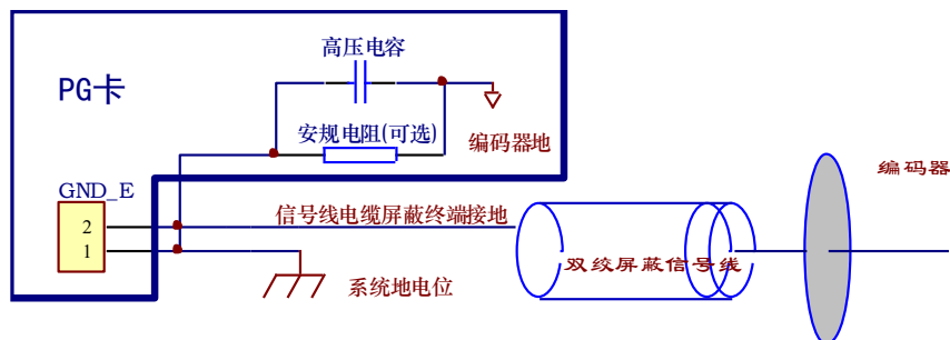
图 3.17 SPG_V6 / SPG_V6D 接口卡连接示意图
