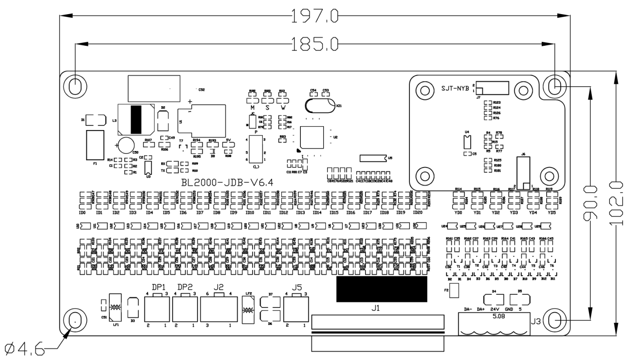
图 11.10 BL2000-JDB-V6.4 轿顶板器件位置及尺寸图
