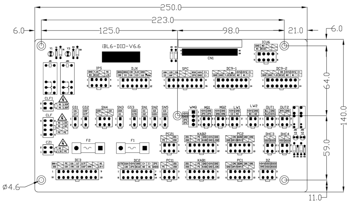
图 11.4 iBL6-DIO-V6.6 轿顶接口板实物图及尺寸图
