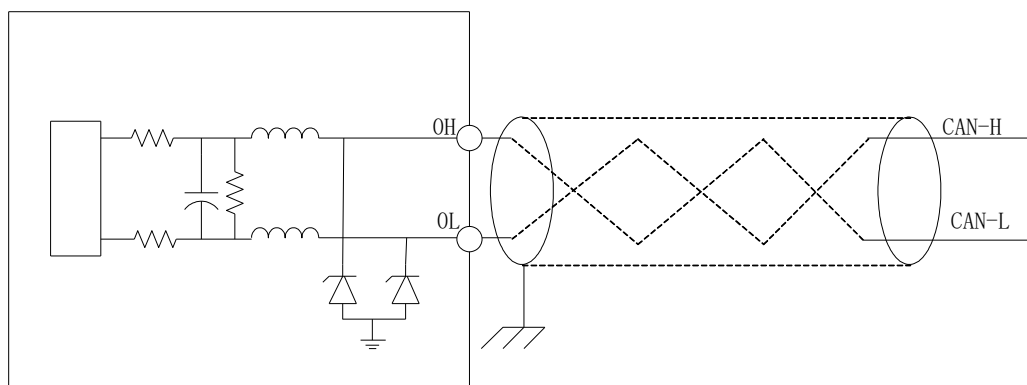
图 3.7 CAN 接口原理及接线示意图
