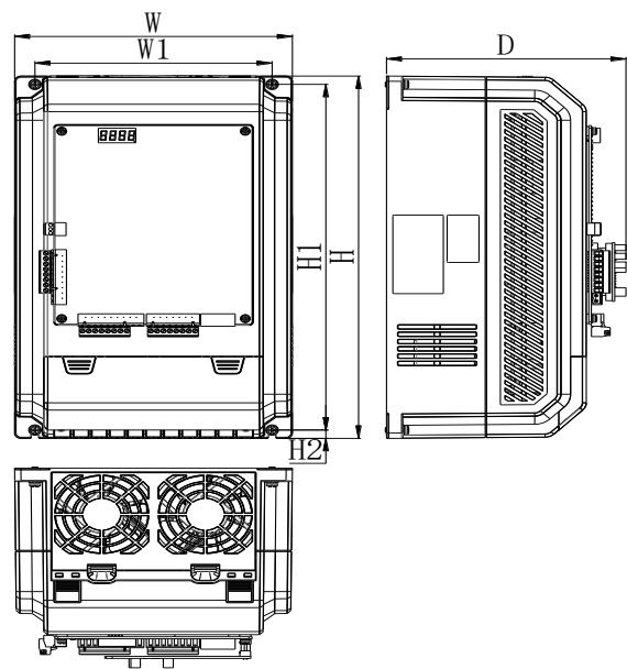
图 2.11 安装尺寸示意图
