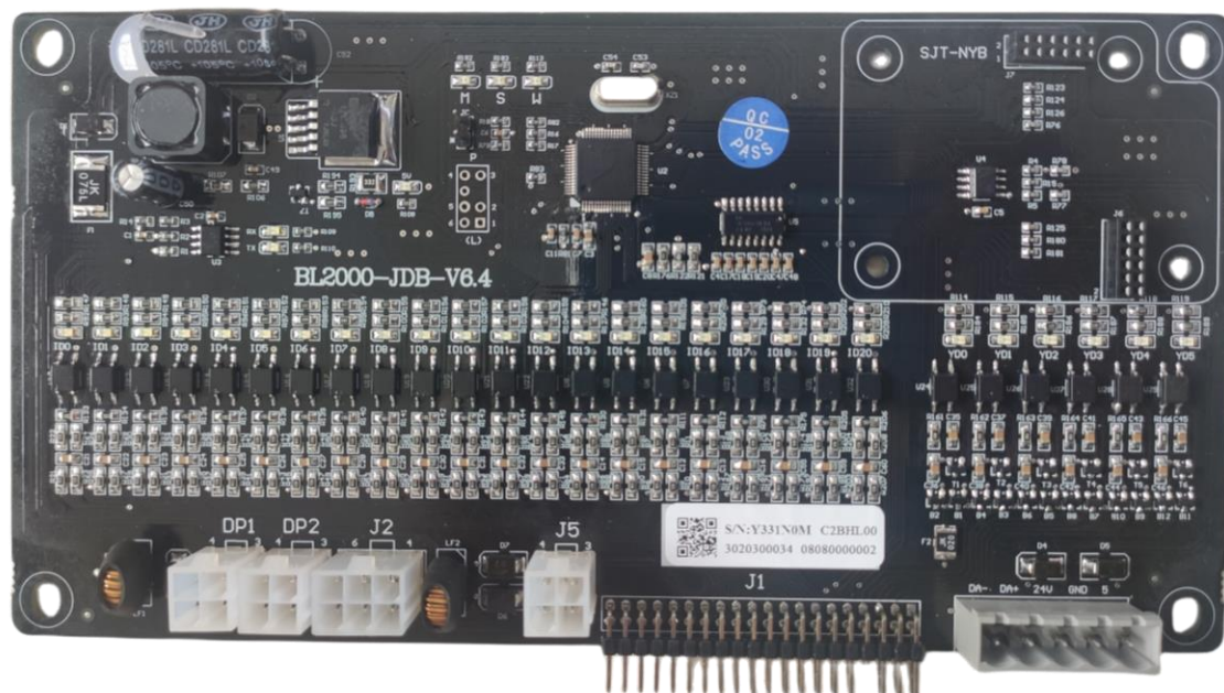
图 11.9 BL2000-JDB-V6.4 轿顶板实物图
