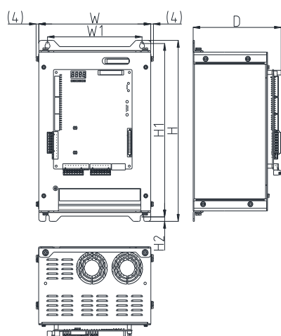
图 2.7 无面板安装尺寸示意图
