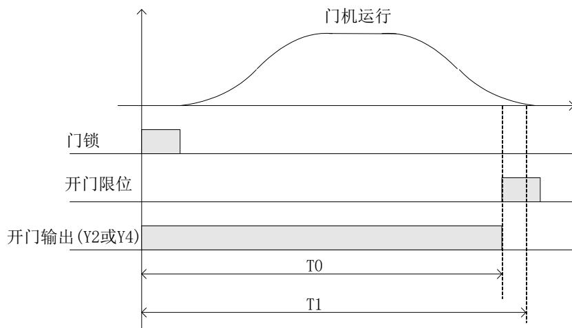
图 6.7 开门时序图
