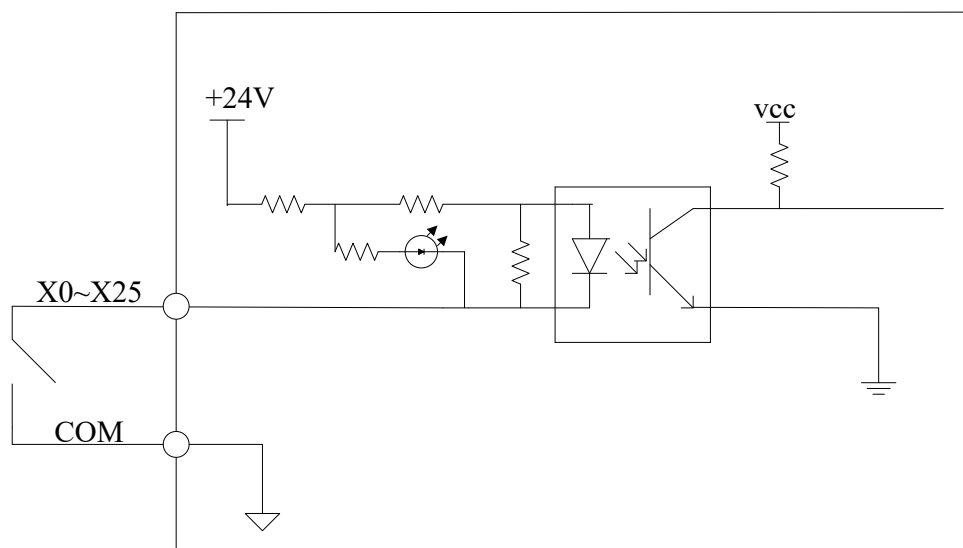
图 3.6 触点开关输入示意图
