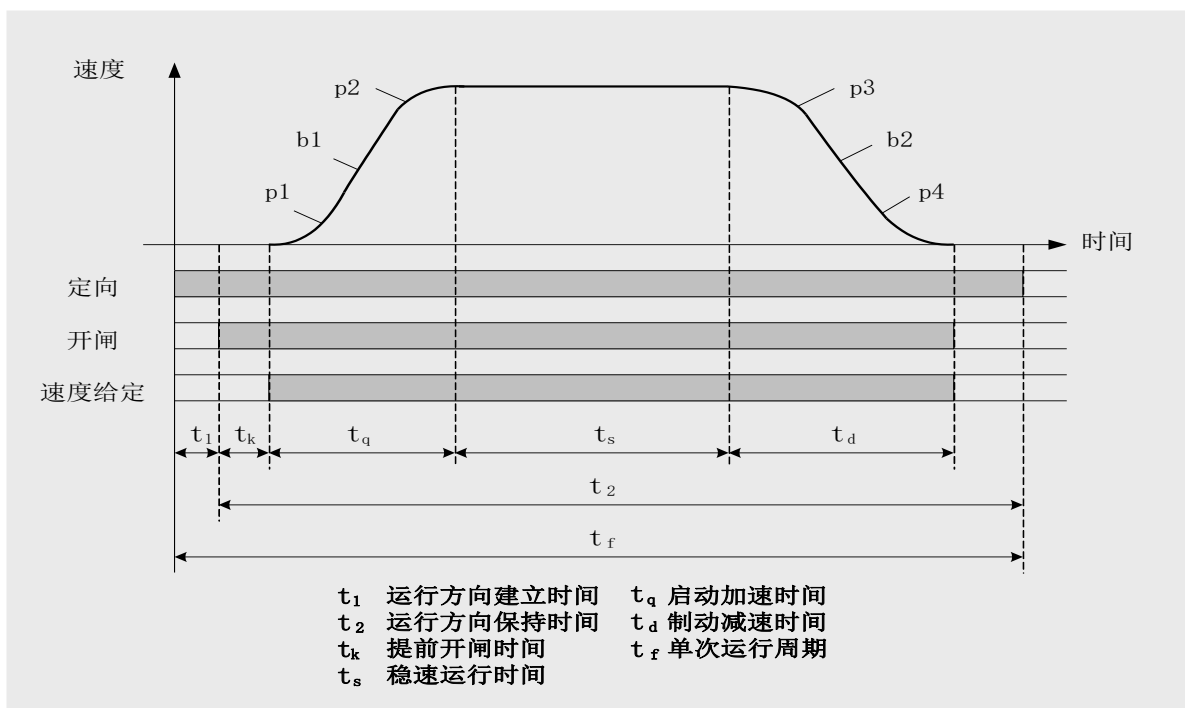
图 7.5 运行曲线图示
