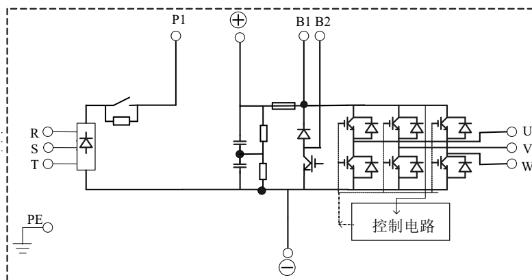
图 3.2 主回路结构示意图
