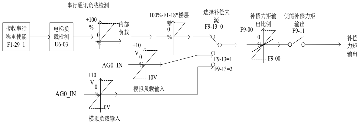
图 6.14 负载补偿力矩输出控制示意图
