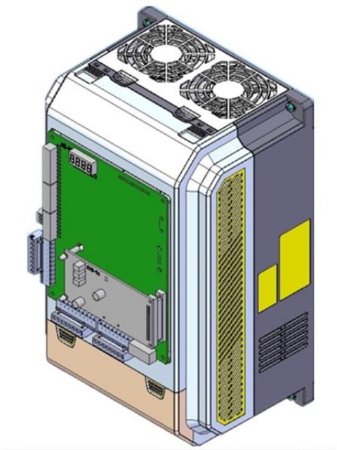
图 2.12 安装外形图
