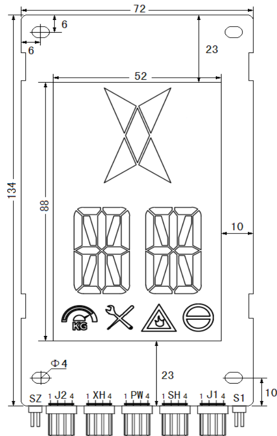
正面尺寸图
