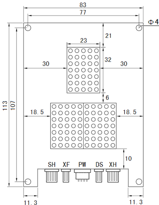
正面尺寸图
