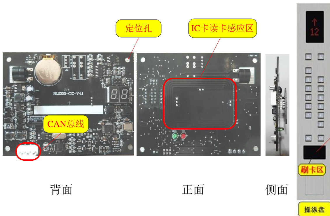
图 2.1 电梯轿厢端控制器 BL2000-CIC-V4.1 实物图
