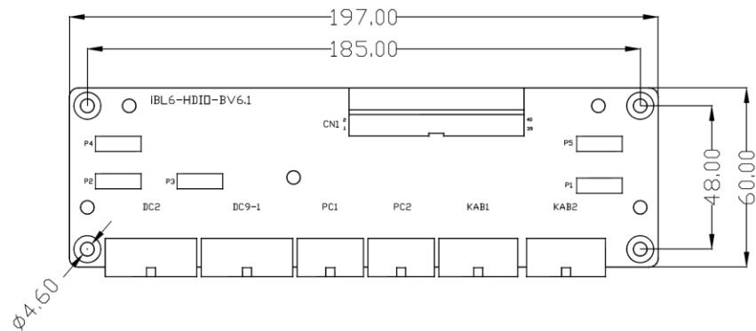
图 2.12 iBL6-HDIO-BV6.1 布局尺寸图
