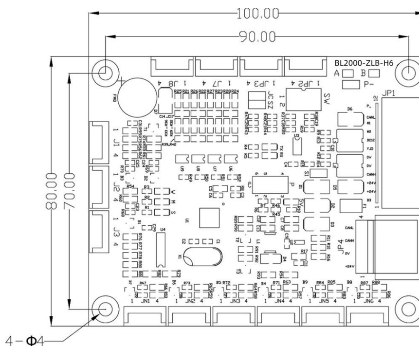
图 2.16 BL2000-ZLB-H6 尺寸布局图
