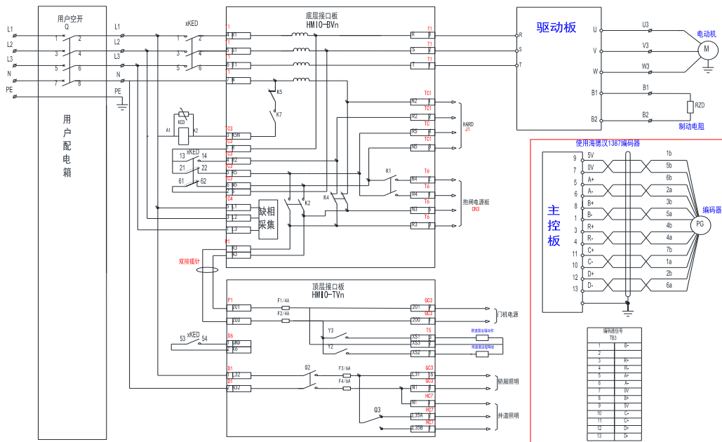
图 3.5 主回路原理图
