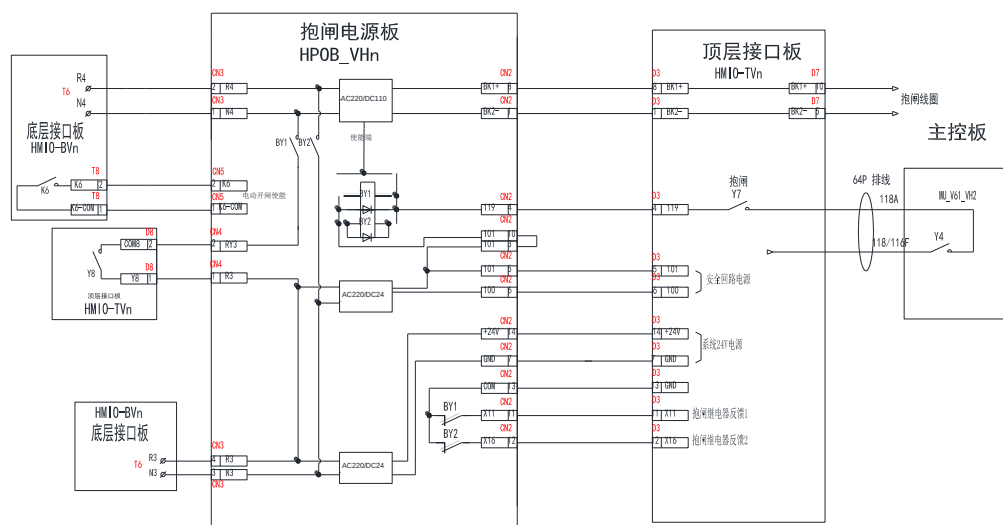
图 3.4 抱闸回路原理图
