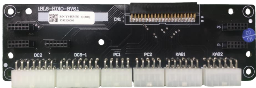
图 2.11 iBL6-HDIO-BV6.1 实物图
