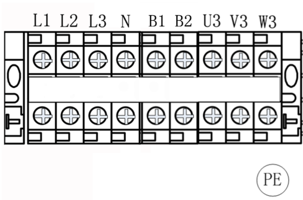
图 3.1 主回路端子示意图
