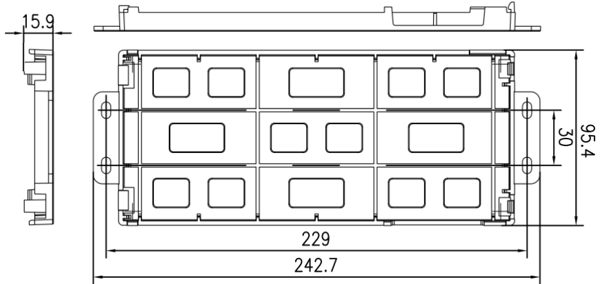
图 2.3 模块化指令板 BL2000-ZLB-V6.X 衬板安装尺寸图
