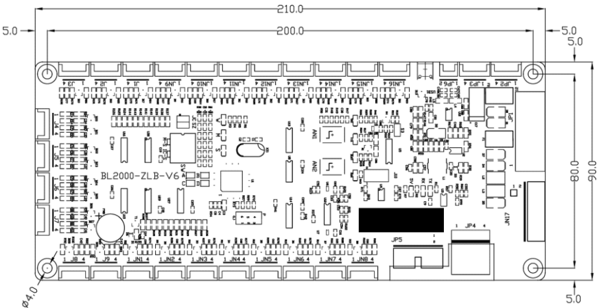
图 2.2 模块化指令板 BL2000-ZLB-V6.X 尺寸图
